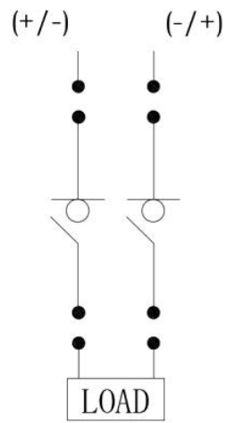
接线图 2 2P 外形
